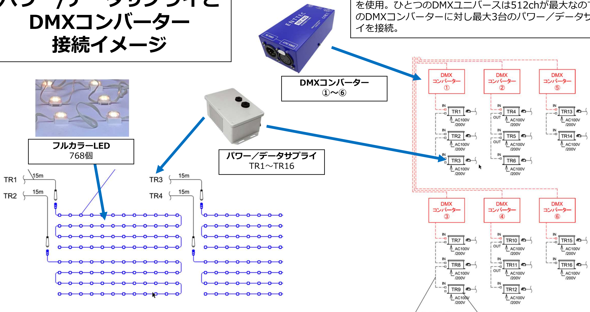
フルカラーLEDとパワー/データサプライの接続イメージ
